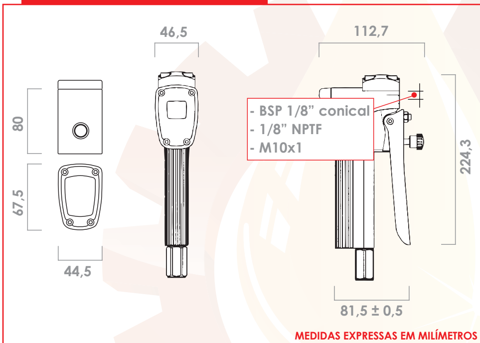
VISOR MULTIFUNÇÃO
