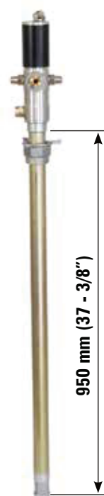
Tambor de 200 Litros MIX-11PT3
