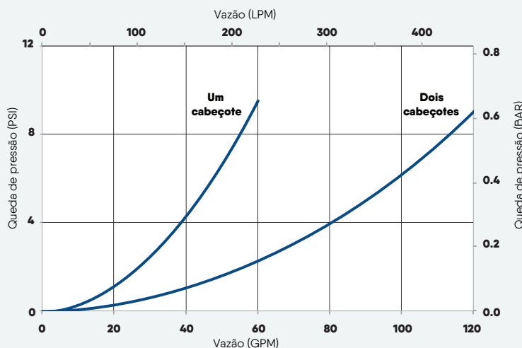
Queda de pressão das cabeças de filtro
