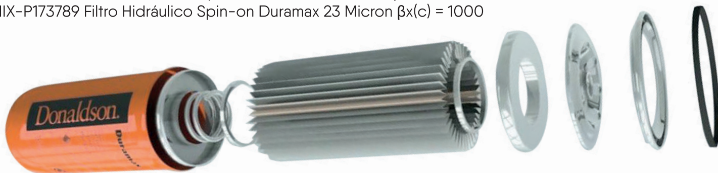
Filtro Donaldson β1000
